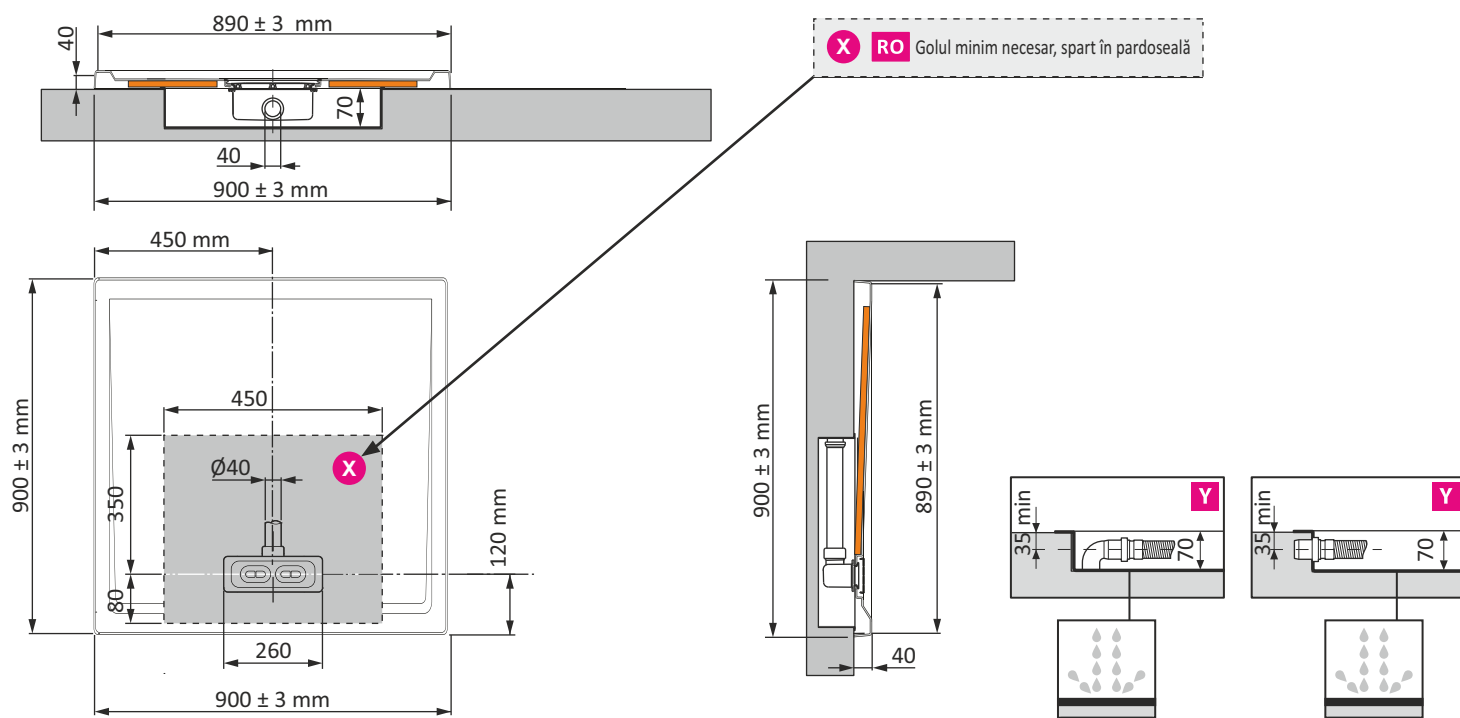
Fig.2 Spargerea și săparea volumului necesar montării sifonului
