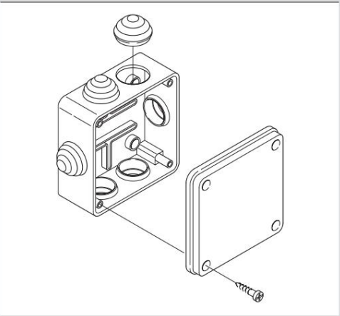
Cutie de jonctiune pentru montare la suprafață 100x100 mm. Cutie de 50 mm înălțime cu manșoane pentru cablu IP55. Capac închis cu șuruburi.
