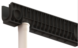
Conexiune verticală
