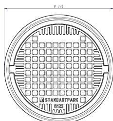
Schita vedere superioara
