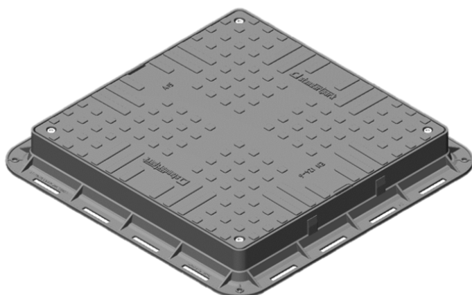
Capac PP URBAN Negru patrat necarosabil 700x700 PL.550x550 Hext.80 cu 4 inchizatoare A15 (35487-20)
