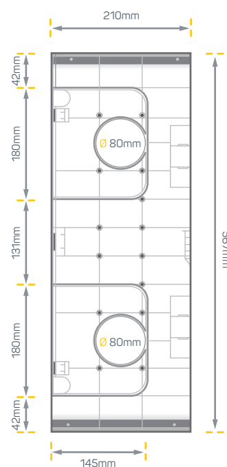
Fig. 4 Perete lateral
