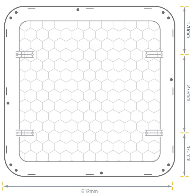
Fig. 3 - Panou ancorare
