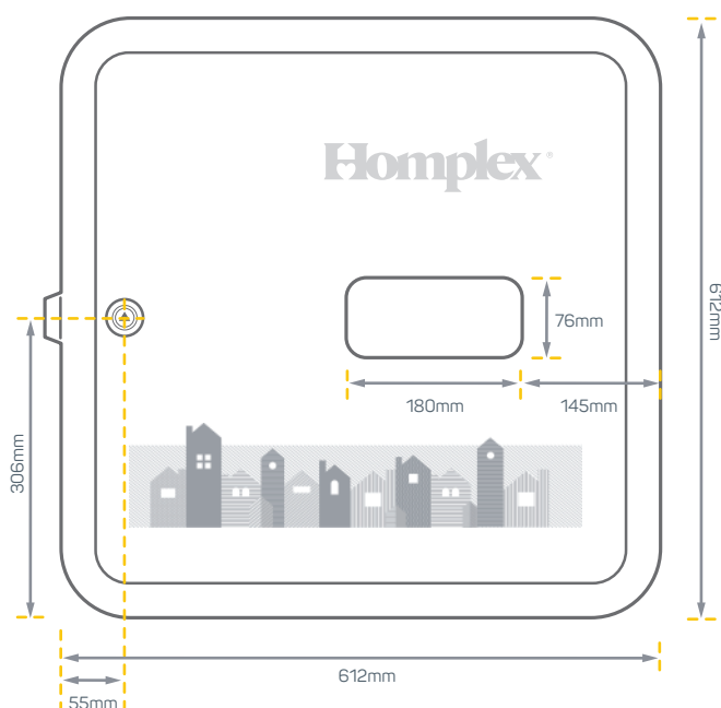
Fig. 3 - Panou ancorare
