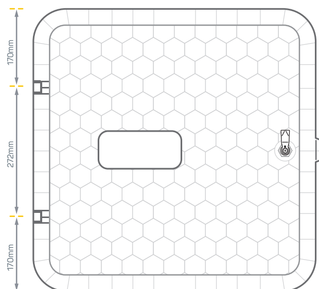
Fig. 2 - Ușă, vedere verso
