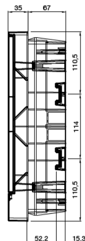
Montat încadrat
