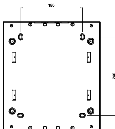
Montat aparent
