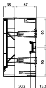
Montat aparent
