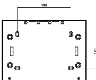
Montat aparent
