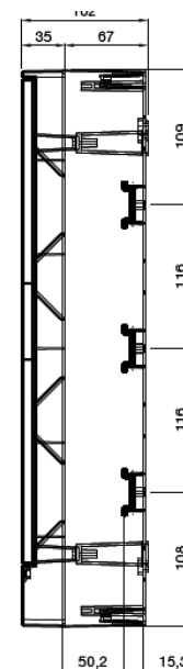
Montat aparent
