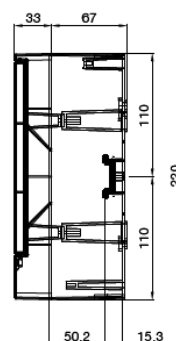
Montat aparent
