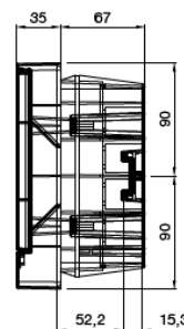
Montat încadrat
