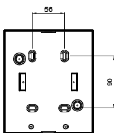
Montat aparent
