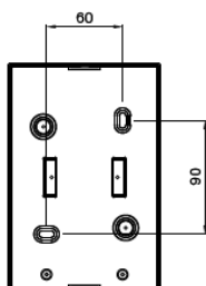
Montat aparent
