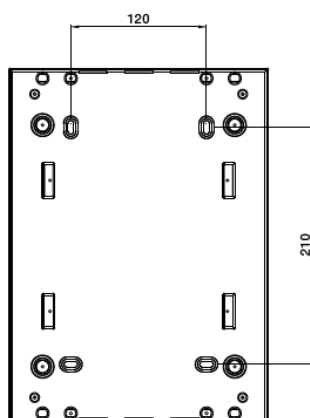
Montat aparent
