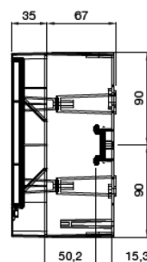
Montat aparent
