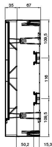
Montat aparent
