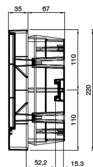
Montat încadrat
