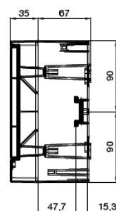
Montat aparent
