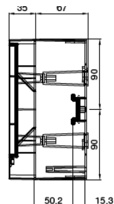
Montat aparent
