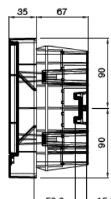
Montat încadrat
