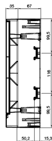
Montat aparent
