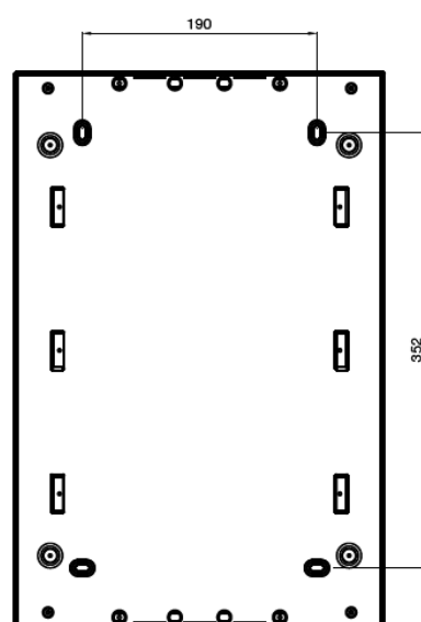
Montat aparent
