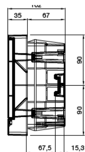
Montat încadrat
