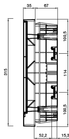
Montat încadrat
