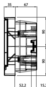
Montat încadrat
