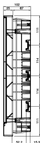
Montat încadrat
