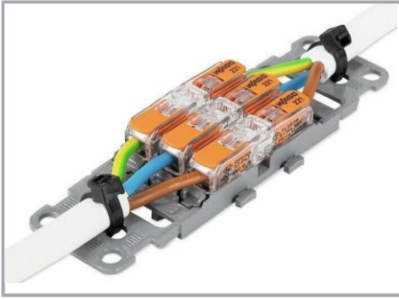
Adaptor de ȳrindere 3-polar cu protecție contra tensiunilor mecanice
