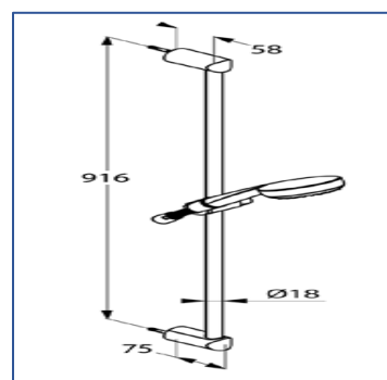
Schiță tehnică
