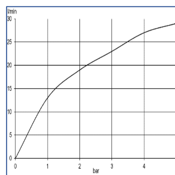
Diagramă de debit
