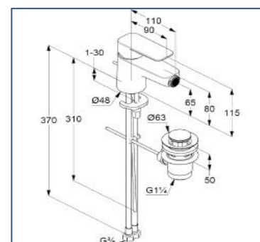
Schiță tehnică
