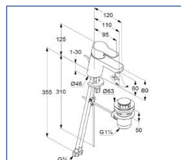
Schiță tehnică
