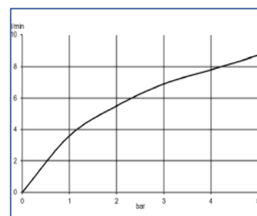
Diagramă de debit
