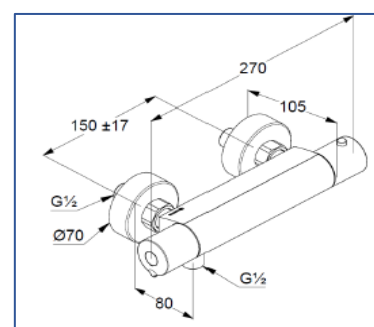
Schiță tehnică
