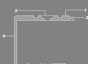
Scara 1:1 ATP257
