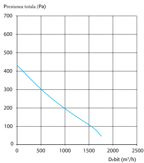
- Canal Fast 315
