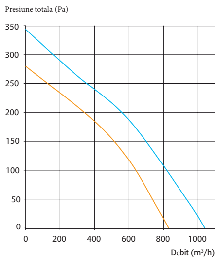
- Canal Fast 200
