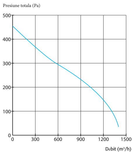
- Canal Fast 250
