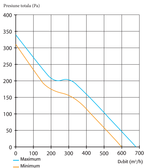
- Canal Fast 315
