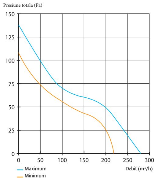
- Canal Fast 160
