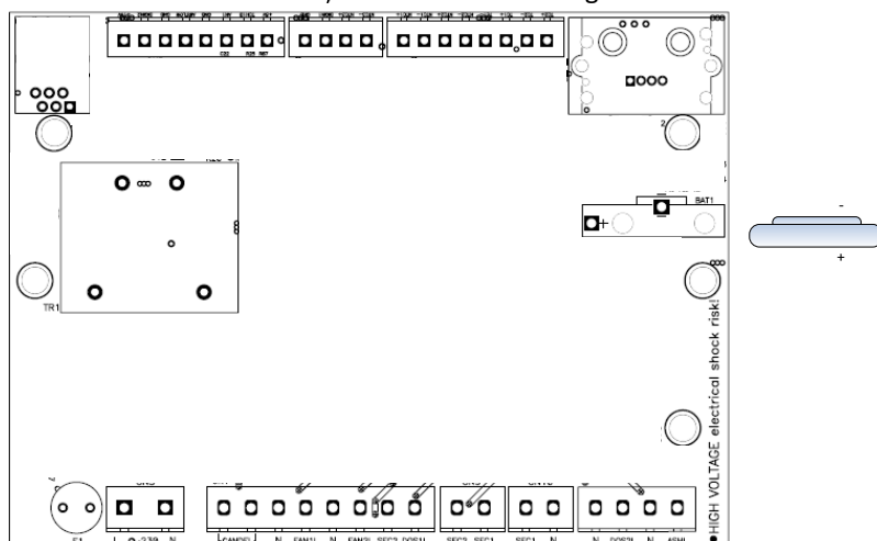
Figura 4: Inlocuirea bateriei
