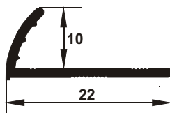
ERT107
