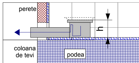
Fig.5 cazul I – Montarea unui sifon plat care se incadreaza in distanta ( h ) dintre gura de scurgere a caditei si pardoseala.
