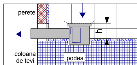
Fig.6 cazul II – Montarea unui sifon plat care nu se incadreaza in distanta ( h ) dintre pardoseala si gura de scurgere a caditei, necesitand crearea unui spatiu in pardoseala, permitand montarea sifonului.
