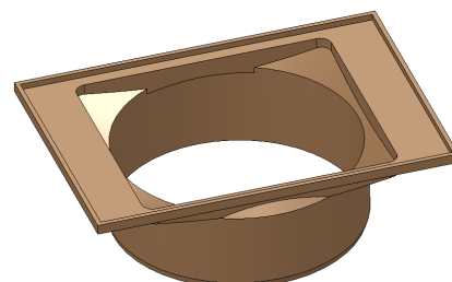
Fig. 2 Piesa de sprijin pentru gratar fonta clasa C250
