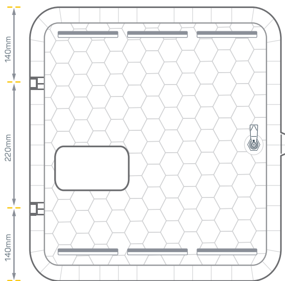
Fig. 2 - Ușă, vedere verso
