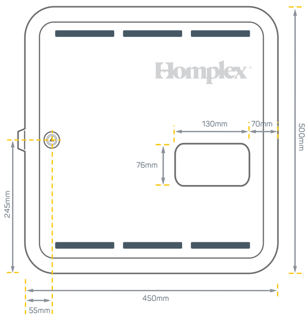
Fig. 3 - Panou de ancorare
