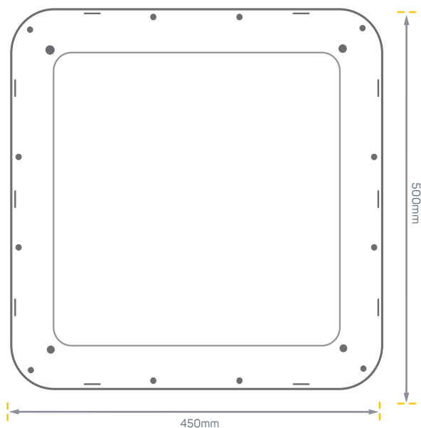
Fig. 3 - Panou de ancorare
