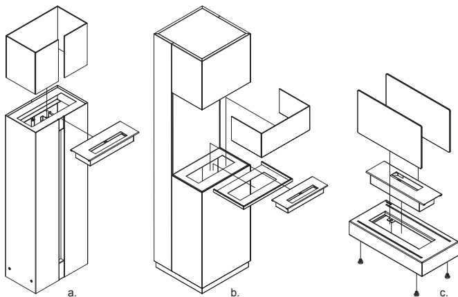
Rys. 7. Montajul gamei: a) Romeo, b) Sierra, c) Galina d) Hotel S
