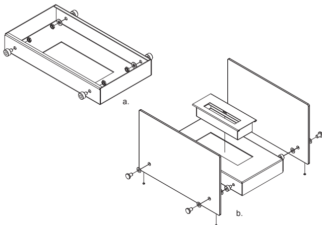
Fig. 5. Montajul Biosemineelor din seria HOTEL
