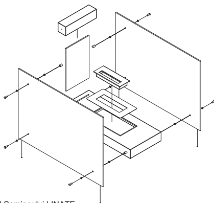
Rys. 6. Montajul Semineului LIMATE
