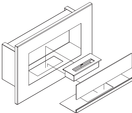
Rys. 8. Montajul sticlei decorative pe baza metalica. Exemplificat pe modelul Delta
