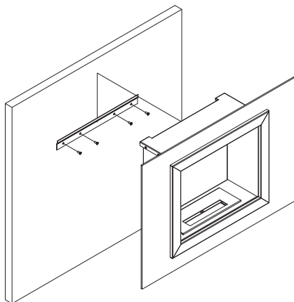
Fig. 4. Montajul Biosemineelor de tip OSCAR
