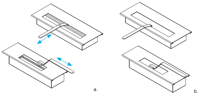
Fig. 2. Exemple de rezervoare de biocombustibil cu capac culisant: (a) deschis; (b) închis
