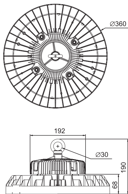
DALI 120W - 200W
