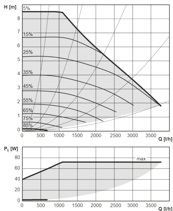
Curbe de putere ale pompei Wilo Para 25/8 iPWM1
