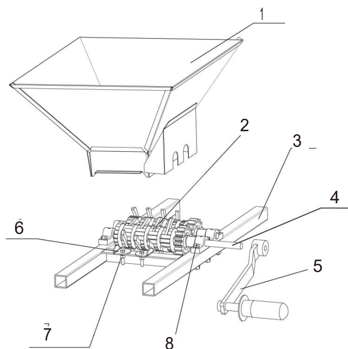
1 – Structură zdrobitor de fructe
