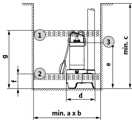
Fig. 2: Димензии на инсталација и точки на прекинување
