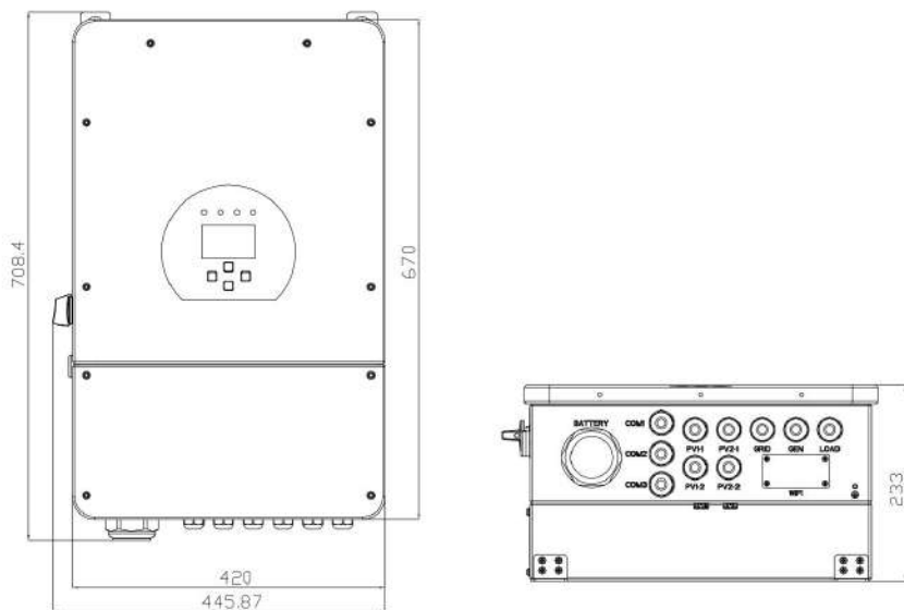
Dimensiunea invertorului
