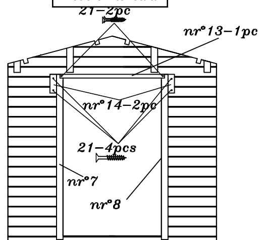
Vedere interioara
