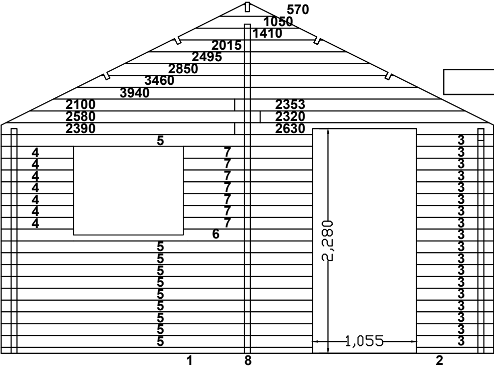
Perete fata, vedere exterioara
