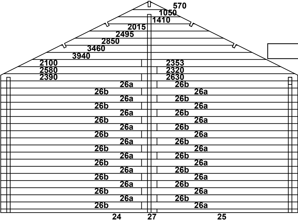
Perete spate, vedere exterioara
