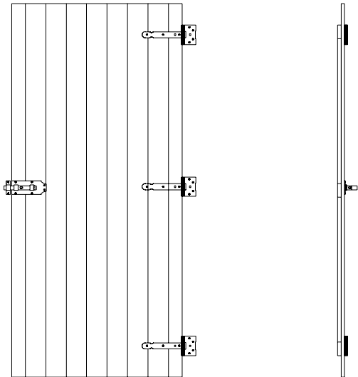
Vedere exteriora
