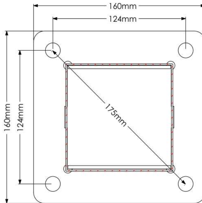
Dimensiunile plăcii de fixare
