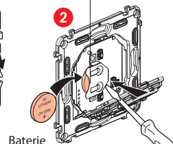
Baterie cu litiu CR 2032 3 V
