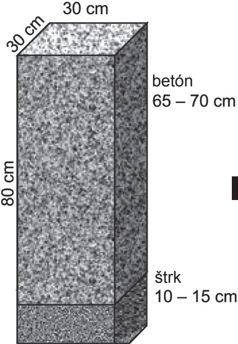
ZÁKLADŇA
