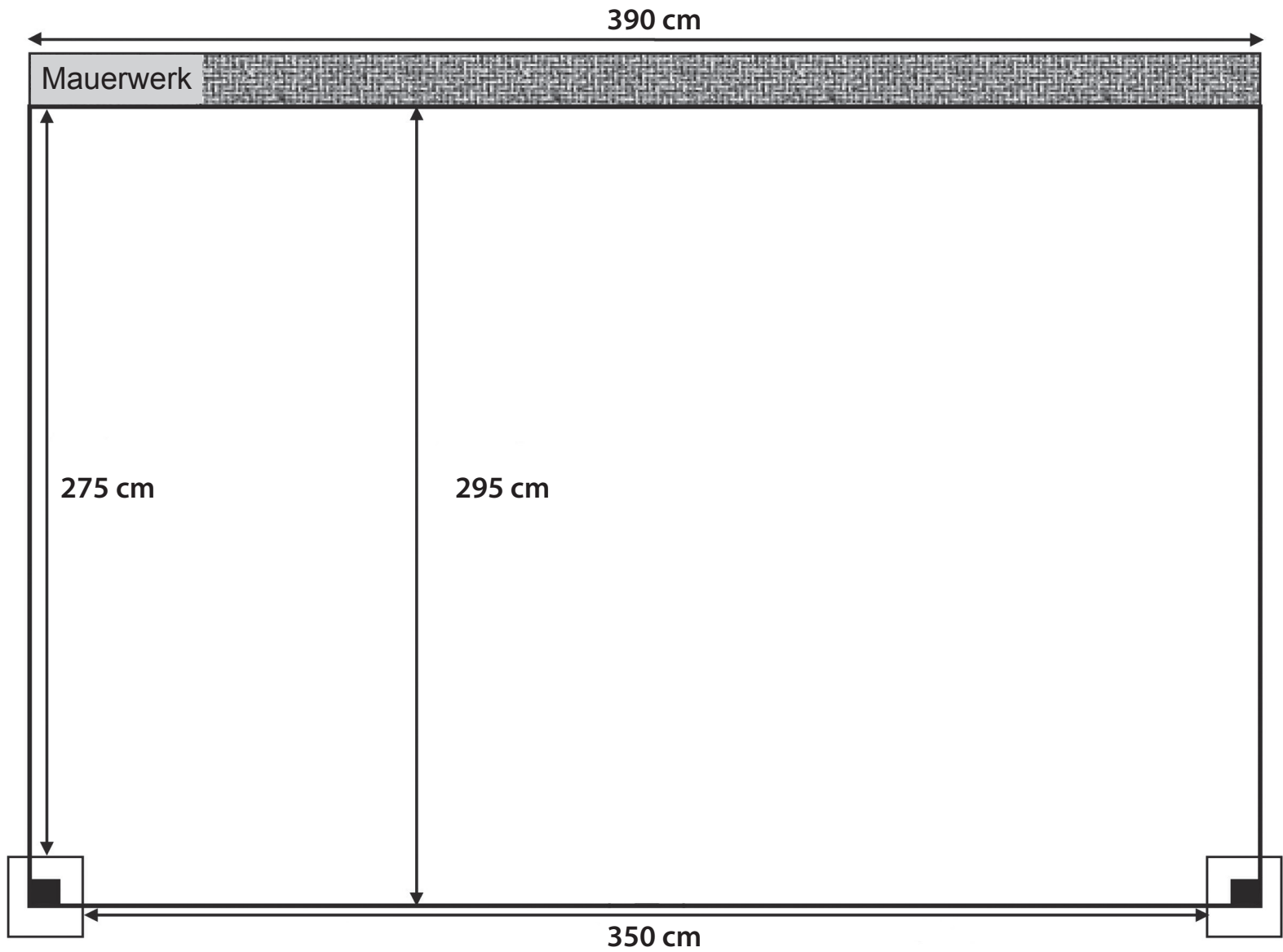
FUNDAMENT
