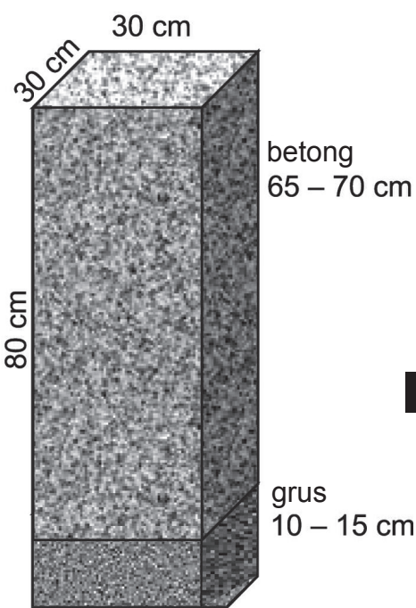
FUNDAMENT
