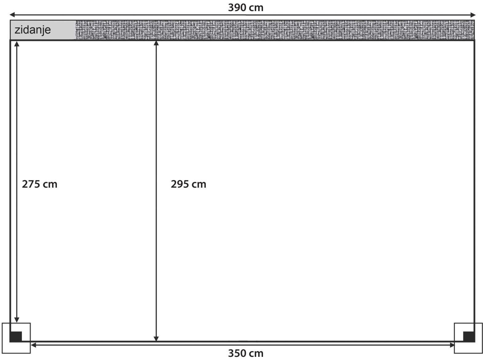
TEMELJ
