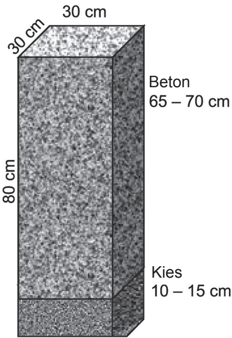
FUNDAMENT
