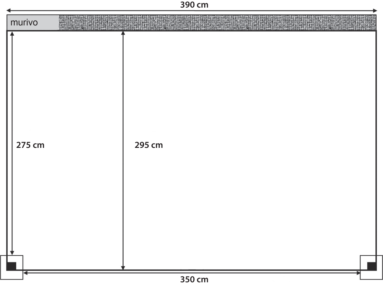
ZÁKLADŇA
