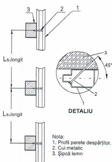
A-A (cu rigidizare pe lemn)
