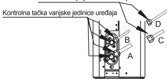
A: Zaporni ventil niskog tlaka B: Zaporni ventil visokog tlaka C & D: Matice unutarnjeg dijela
