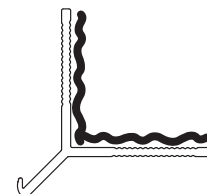
Instalación: Adhesivo
