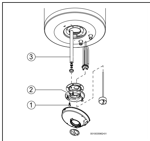
Fig. 14 Accesul la partea interioară și identificarea componentelor
