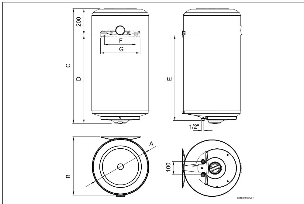
Фиг. 2 Размери в mm (вертикален монтаж)
