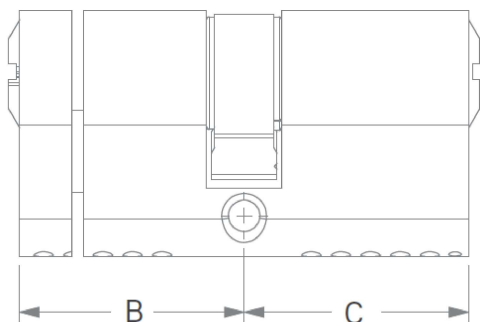
Fig.1 – cilindru dublu cu protecție anti-rupture
