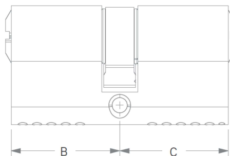
Fig.2 – cilindru dublu
