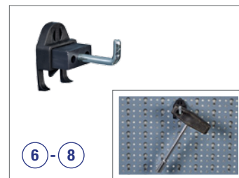
Art.-Nr. 7202-1 (HB-Art. 3205683) 30 mm Art.-Nr. 7202-2 (HB-Art. 3205694) 50 mm Art.-Nr. 7202-3 (HB-Art. 3205707) 60 mm Câte 5 bucăți – pentru role de bandă adezivă, filiere, inele, chei, șaibe, foarfece, etc.
