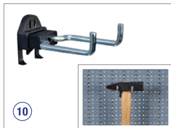
Art.-Nr. 7204 (HB-Art. 3205729), 4 bucăți Lungimea cârligelor 60 mm Distanța 35 mm De exemplu pentru ciocane, etc.
