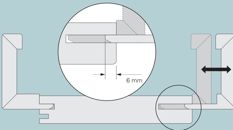
Secțiune transversală: Comparatie între variantele de toc de ușă vechi și noi
