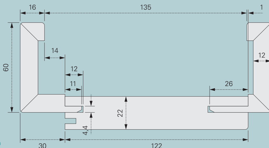
Geometria tocului de ușă pentru o grosime a peretelui de 140 mm (dimensiuni în mm)
