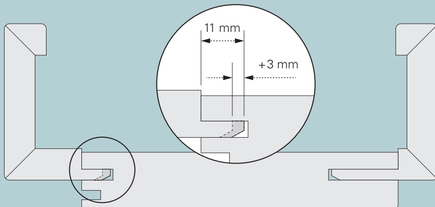
Secțiune transversală: Comparatie între variantele de toc de ușă vechi și noi
