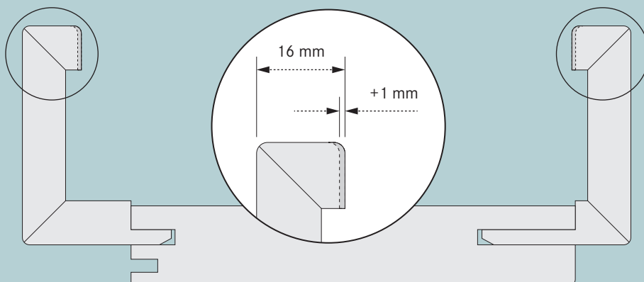
Secțiune transversală: Comparatie între variantele de toc de ușă vechi și noi
