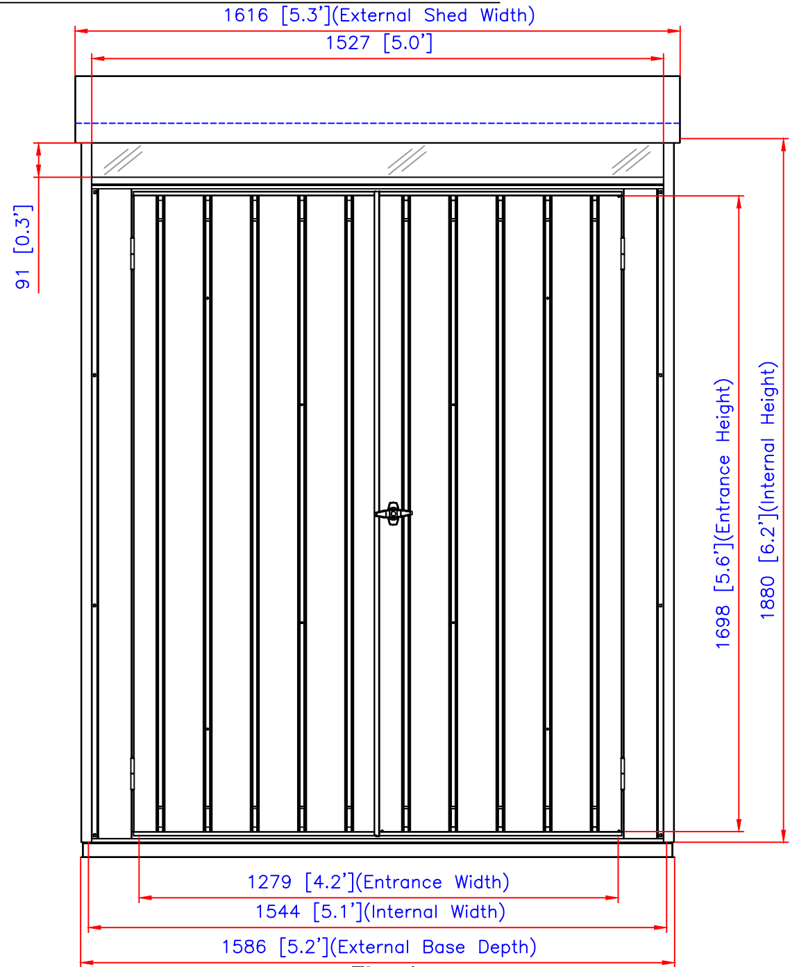
Elevation
