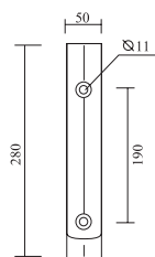
talpă fixare braț
