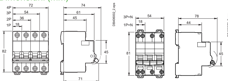
Înteruptor automat 1P, 2P, 3P, 4P
